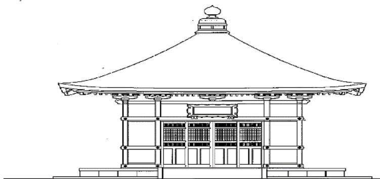
本堂 南立面図 S=1/100
